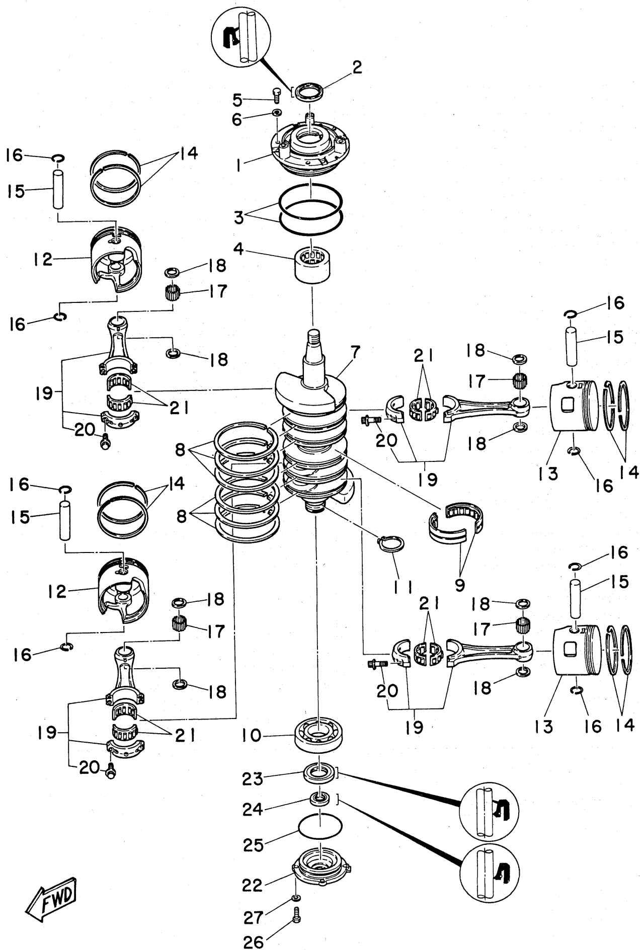
Fig. 2 CRANK & PISTON
